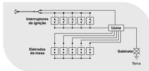
Figura 27 - Diagrama elétrico do acendimento - Cooktop 5 queimadores
