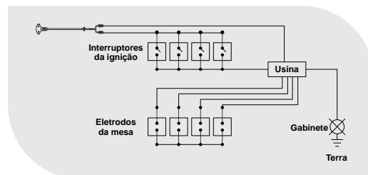
Figura 26 - Diagrama elétrico do acendimento - Cooktop 4 queimadores
