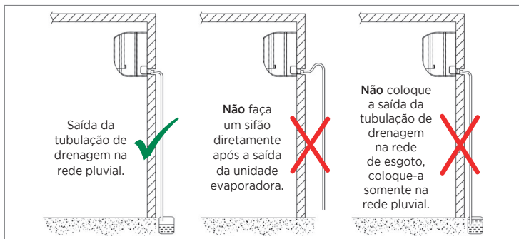
FIG. 7 - EXEMPLOS DE SITUAÇÕES DE DRENAGEM
