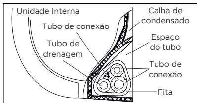
FIG. 8 - TUBO DE CONEXÕES
