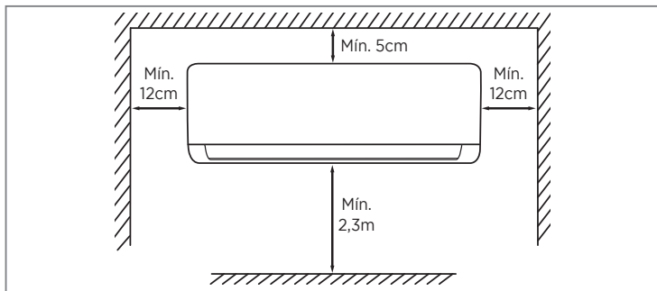
FIG. 6 - ESPAÇAMENTOS MÍNIMOS RECOMENDADOS
