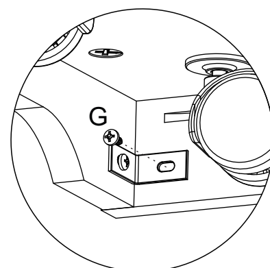
Detalhe 12 Detail/Detalle
