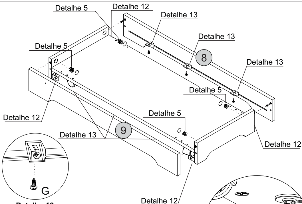
Detalhe 13 Detail/Detalle
